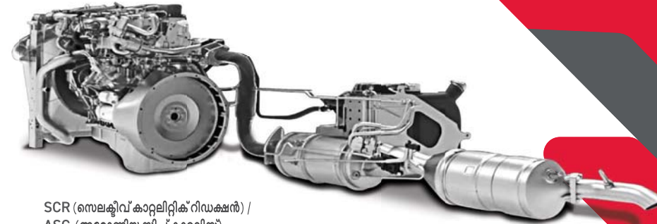
DOC (ഡിസൽ ഓക്സിഡേഷൻ കാറ്റലിസ്റ്റ്) / DPF (ഡിസൽ പാർട്ടികുലേറ്റ് ഫിൽട്ടർ)
