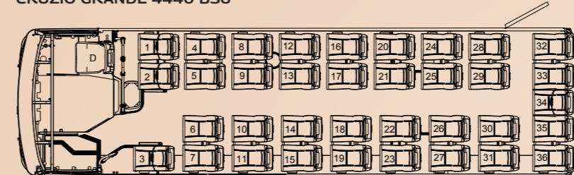
CRUZIO GRANDE 4440 BS6
